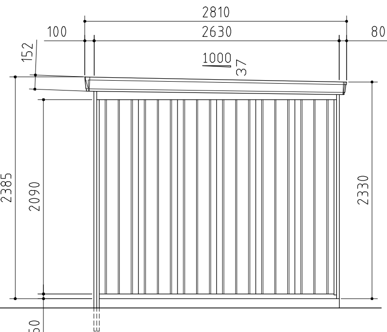
側面図
